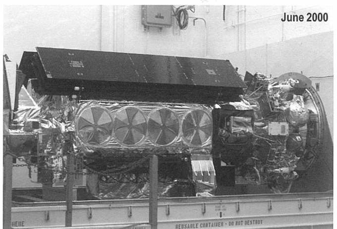
La plataforma NOAA-16, en el laboratorio de pruebas, testeos finales en junio del 2000 antes de ser lanzado al espacio, vector de transporte TITAN II.
